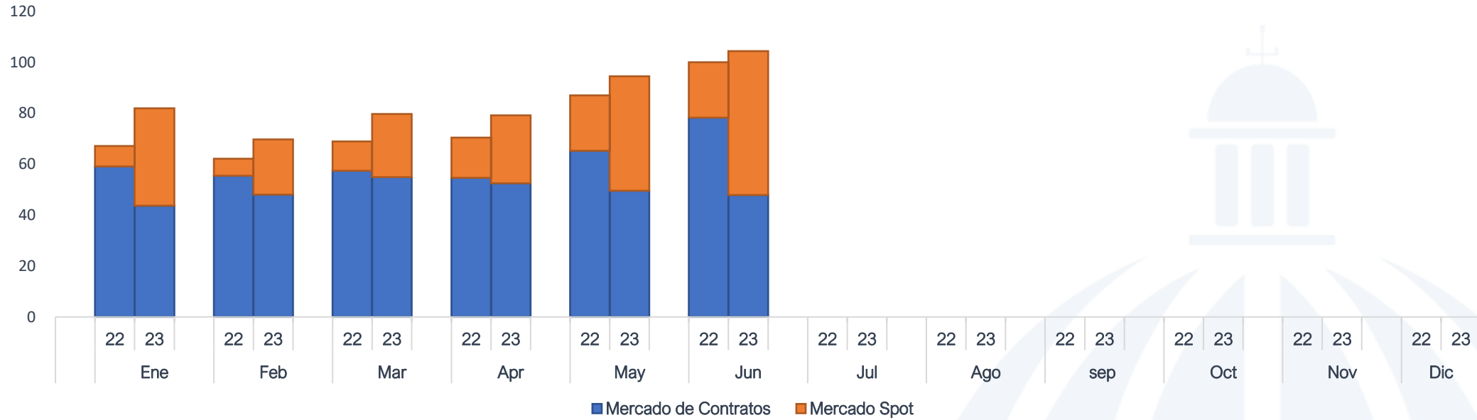
Factura Compra de Energía por Mercado Edesur enero-junio 2023 / enero-junio 2022 (US$ MM)
