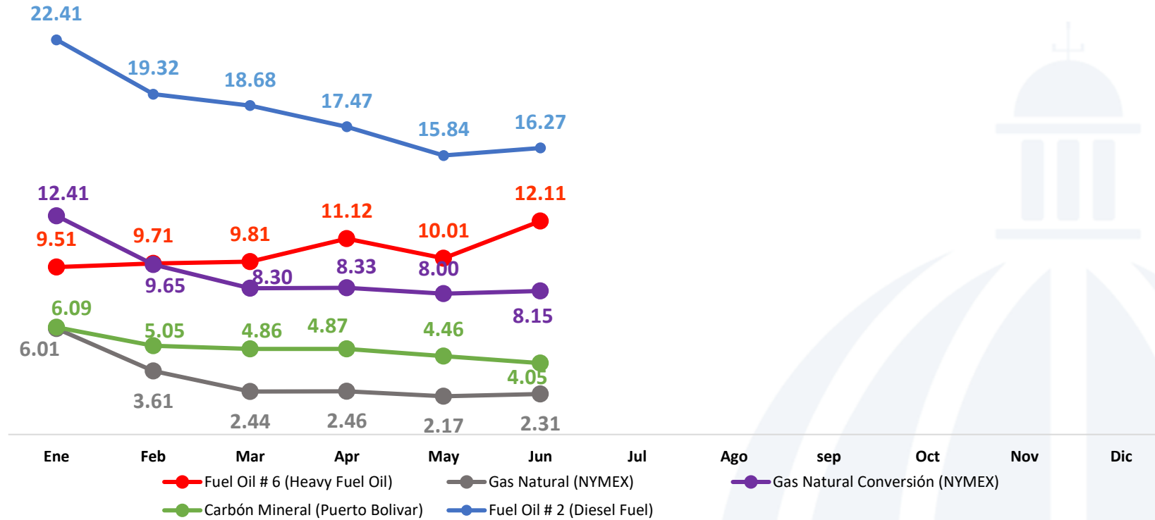
Precio de Combustibles enero-junio 2023 (US$/MMBTU)
