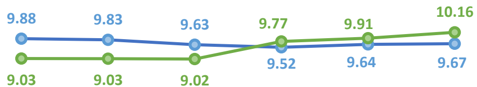
Precio Medio de Venta de Energía Edesur enero-junio 2023 / enero-junio 2022 (RD$/kWh)
