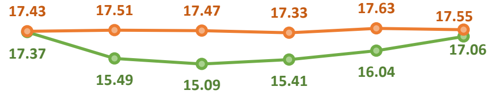
Precio Medio de Compra y Venta de Energía Edesur enero-junio 2023 (USCents/kWh)
