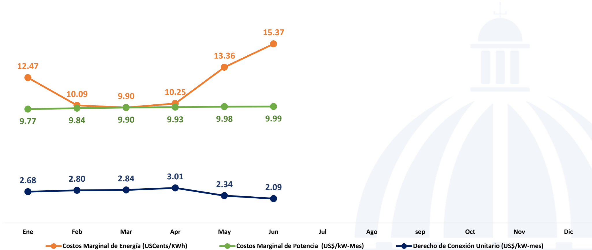
Costos Marginales de Energía, Potencia y Derecho de Conexión Unitario enero-junio 2023 (USCents/kWh y US$/kW-período)
