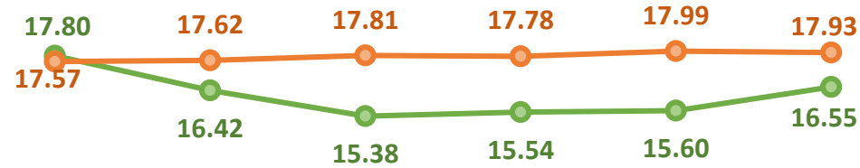
Precio Medio de Compra y Venta de Energía Total EDE's enero-junio 2023 (USCents/kWh)
