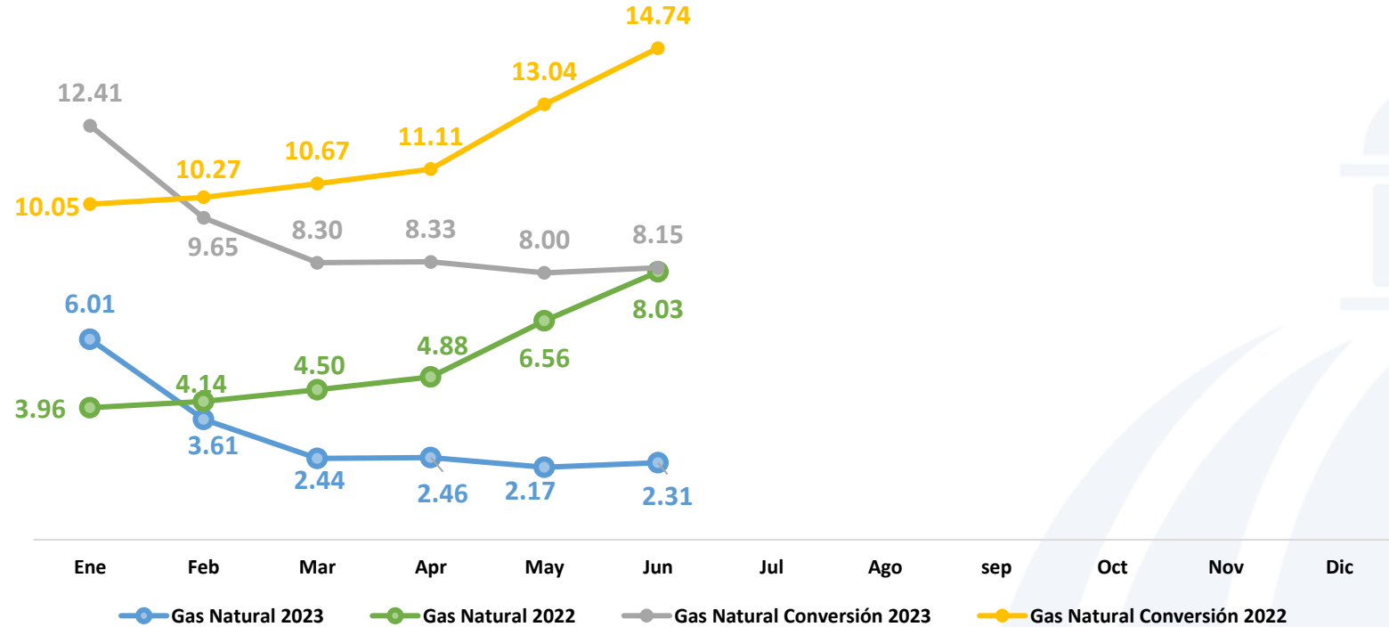
Precio de Combustible Gas Natural enero-junio 2023 / enero-junio 2022 (US$/MMBTU)
