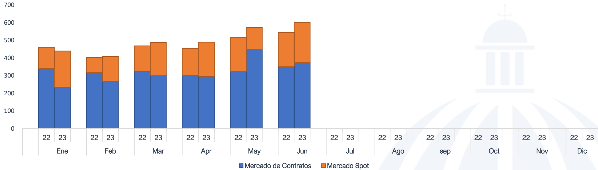
Compra de Energía por Mercado Edeeste enero-junio 2023 - enero-junio 2022 (GWh)
