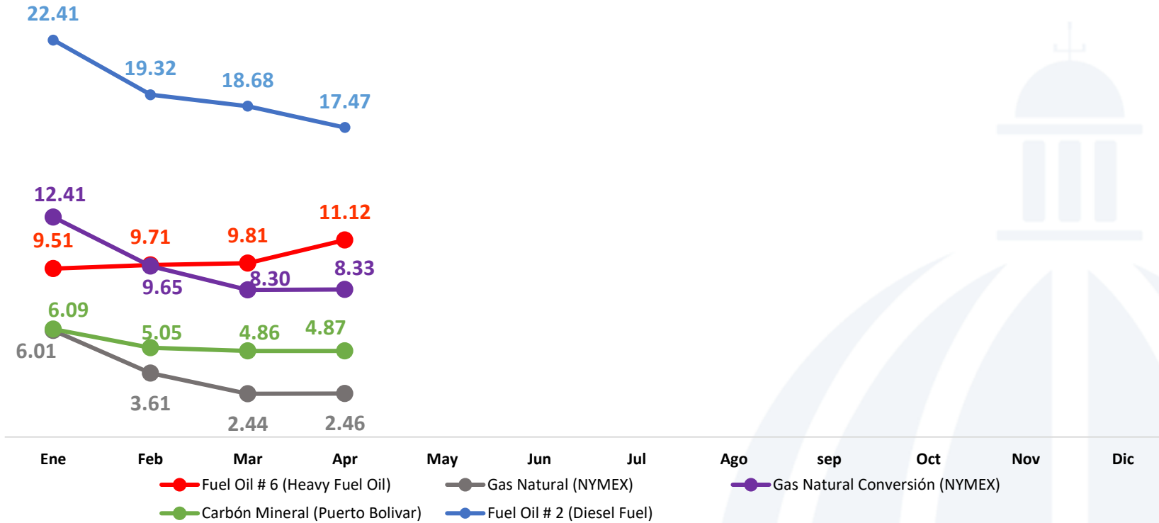
Precio de Combustibles enero-abril 2023 (US$/MMBTU)
