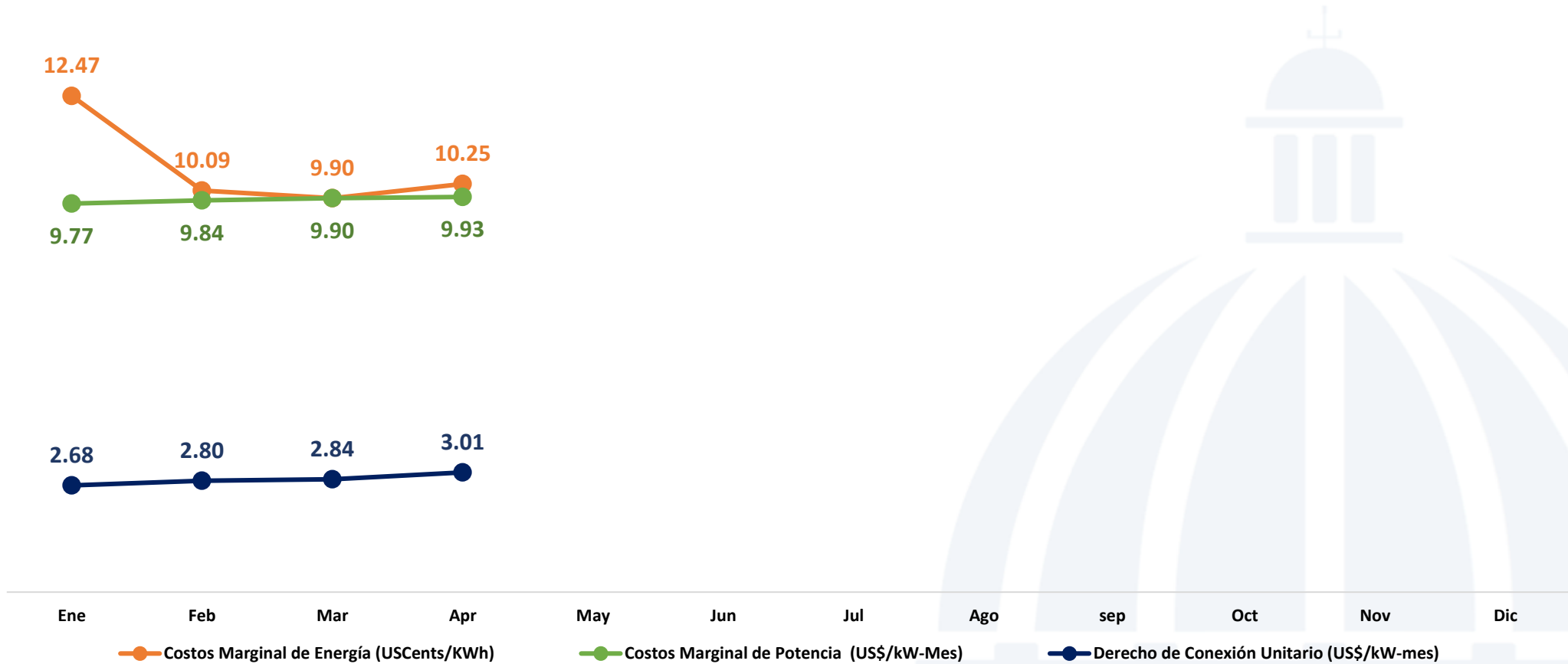
Costos Marginales de Energía, Potencia y Derecho de Conexión Unitario enero-abril 2023 (USCents/kWh y US$/kW-período)
