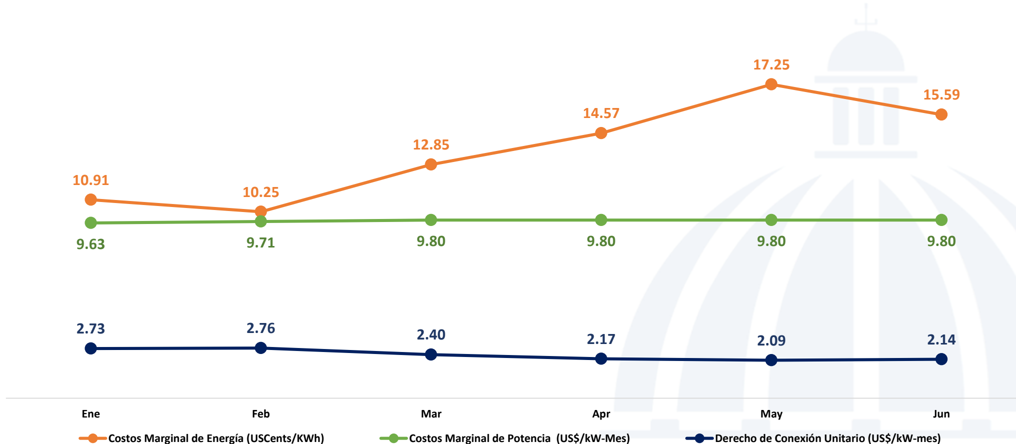
Costos Marginales de Energía, Potencia y Derecho de Conexión Unitario enero-junio 2022 (USCents/kWh y US$/kW-período)
