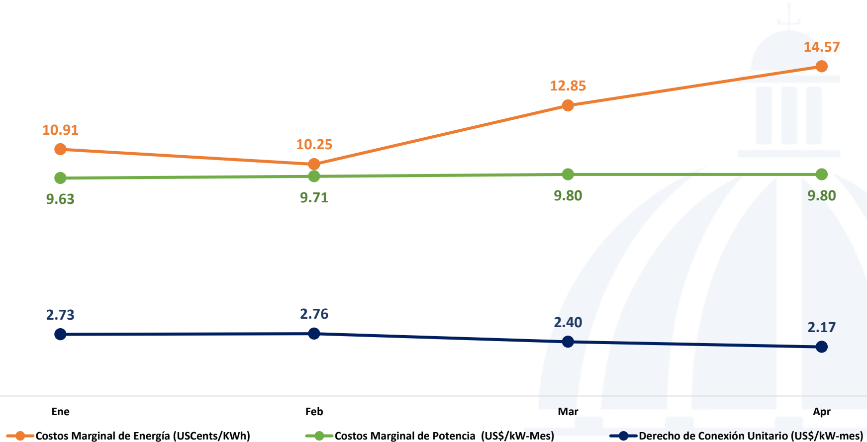
Costos Marginales de Energía, Potencia y Derecho de Conexión Unitario enero-abril 2022 (USCents/kWh y US$/kW-período)
