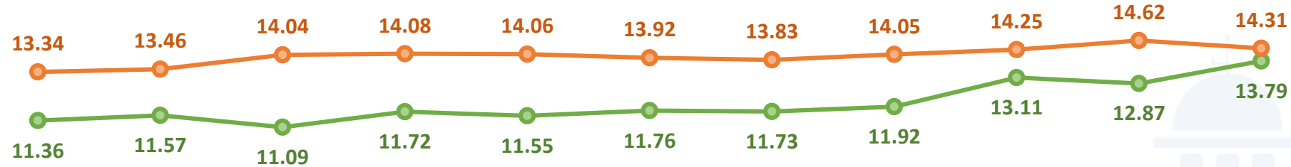
Precio Medio de Compra y Venta de Energía Edeeste ene-nov 2021 (USCents/kWh)
