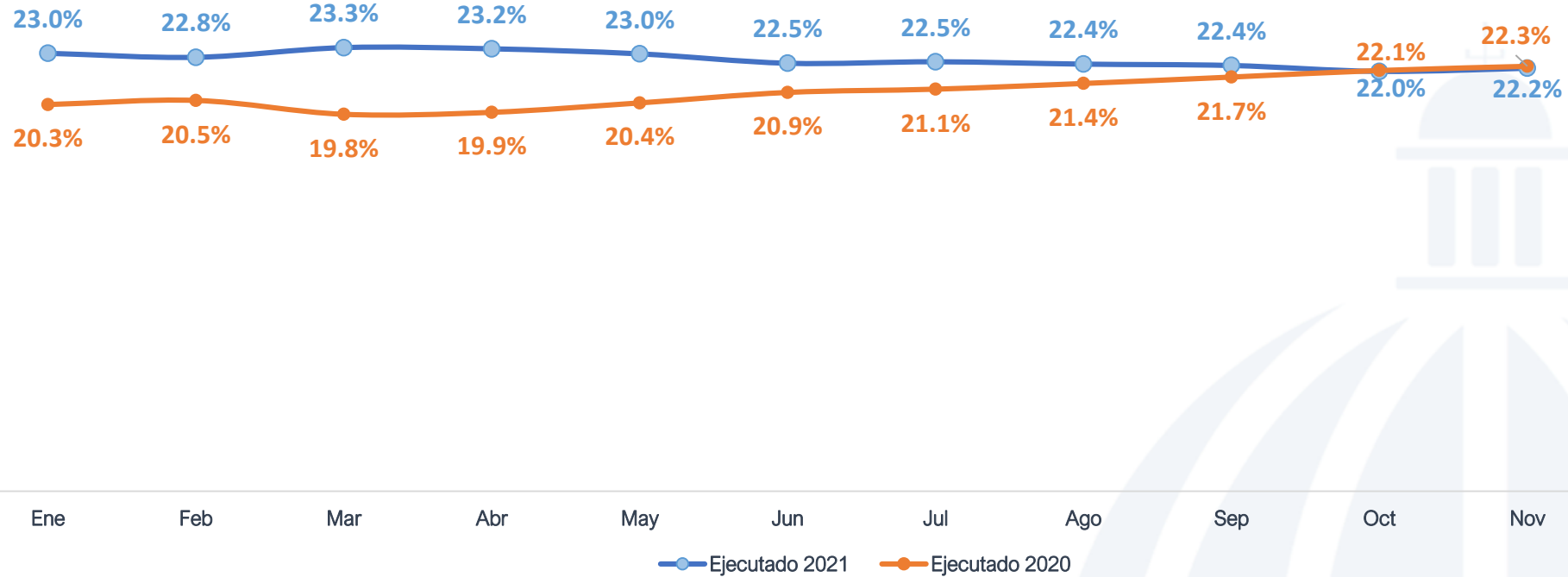
Pérdidas - Año Móvil Edenorte 2021 – 2020 Valores Porcentuales
