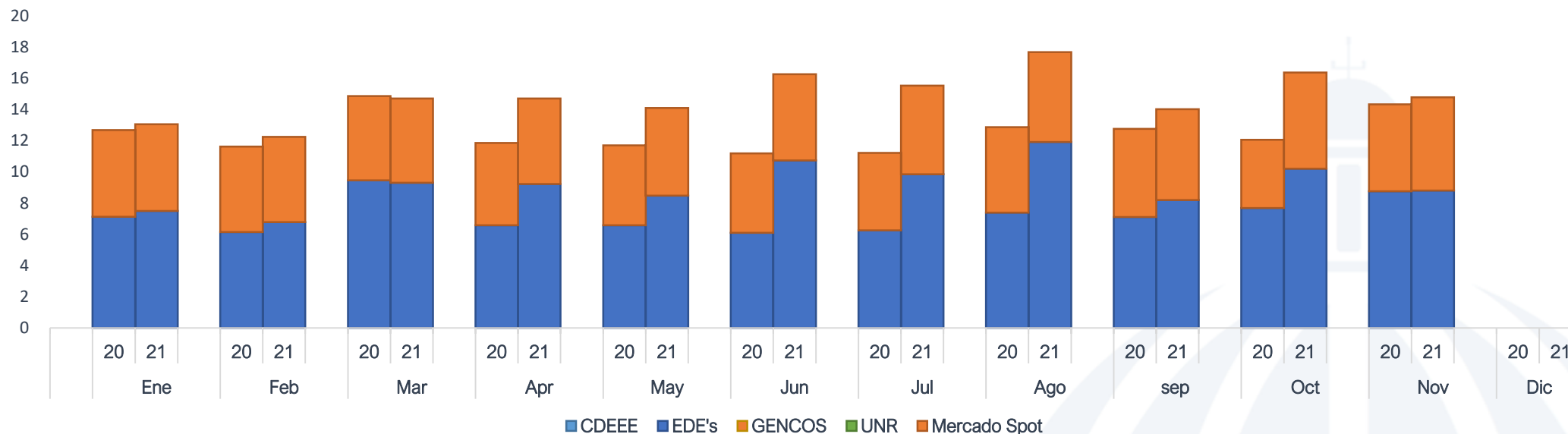
Factura por Venta de Energía EGEHID ene-nov 2021 / ene-nov 2020 (US$ MM)
