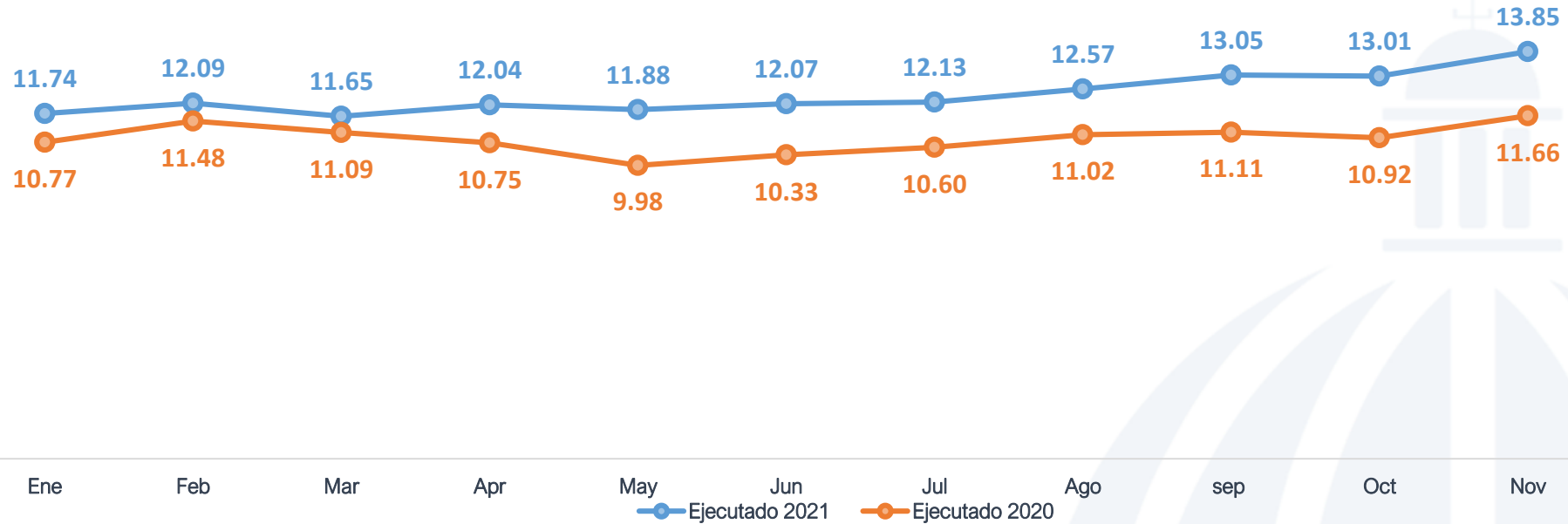
Precio Medio de Compra de Energía Total EDE's ene-nov 2021 / ene-nov 2020 (USCents/kWh)
