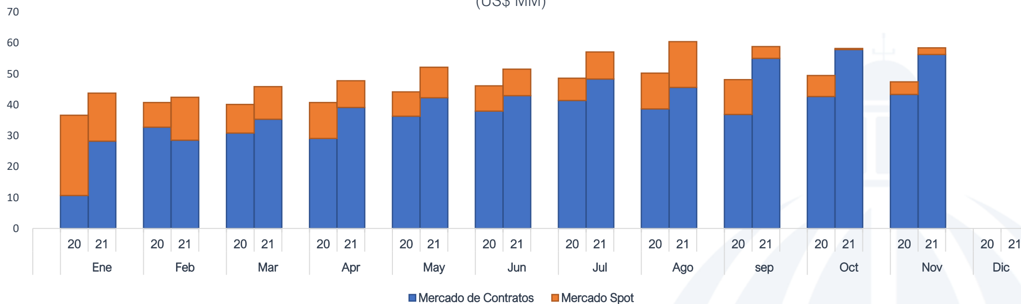
Factura Compra de Energía por Mercado Edenorte ene-nov 2021 / ene-nov 2020 (US$ MM)
