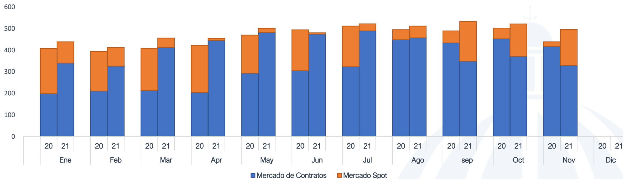
Compra de Energía por Mercado Edeeste ene-nov 2021 / ene-nov 2020 (GWh)
