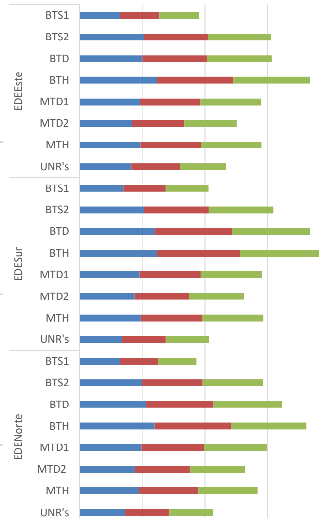
Comparativo Monómico de Ventas por Empresa Distribuidora (RD$/kWh)
