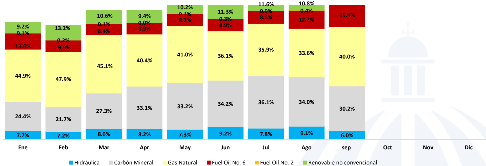
Generación de Energía por Tipo de Combustible enero–septiembre 2021
