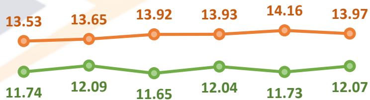
Precio Medio de Compra y Venta de Energía Total EDE's ene-jun 2021 (USCents/kWh)
