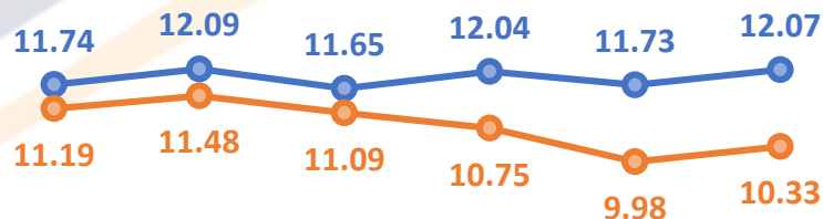
Precio Medio de Compra de Energía Total EDE's ene-jun 2021 / ene-jun 2020 (USCents/kWh)
