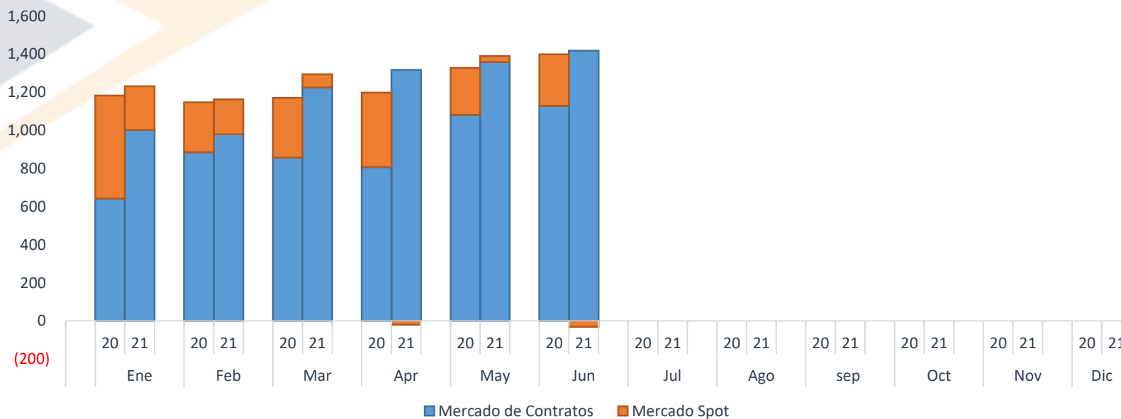
Compra de Energía por Mercado Total EDE's ene-jun 2021 / ene-jun 2020 (GWh)
