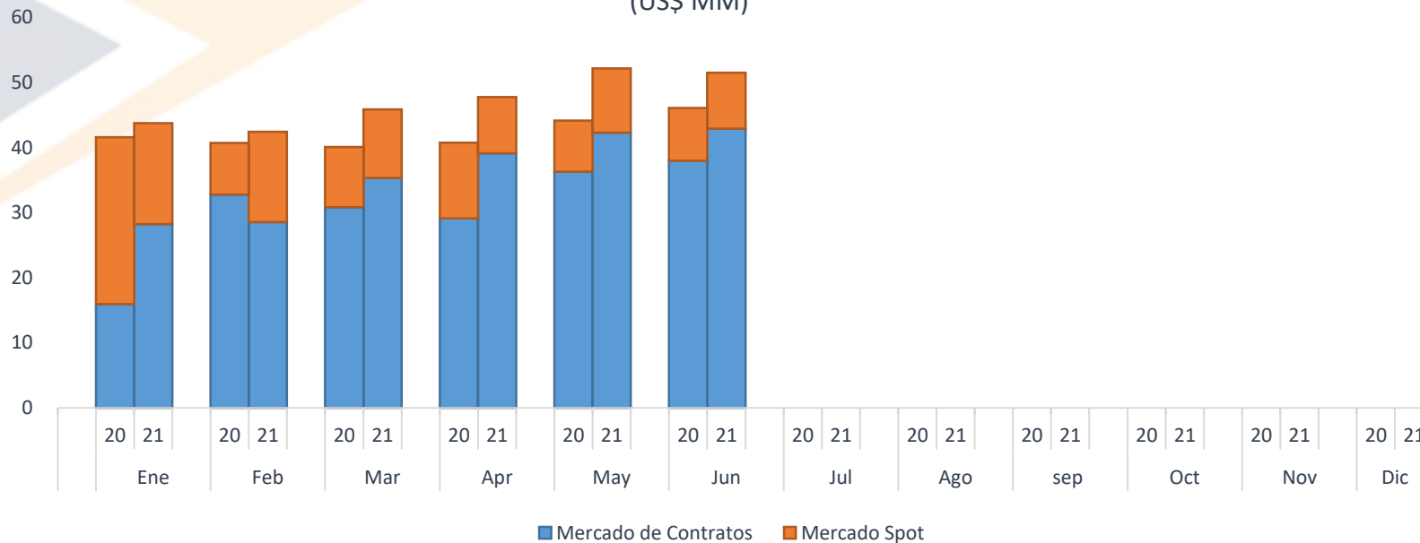
Factura Compra de Energía por Mercado Edenorte ene-jun 2021 / ene-jun 2020 (US$ MM)
