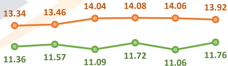
Precio Medio de Compra y Venta de Energía Edeeste ene-jun 2021 (USCents/kWh)
