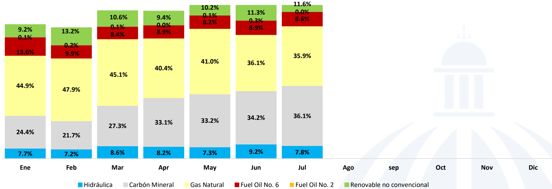
Generación de Energía por Tipo de Combustible enero–julio 2021
