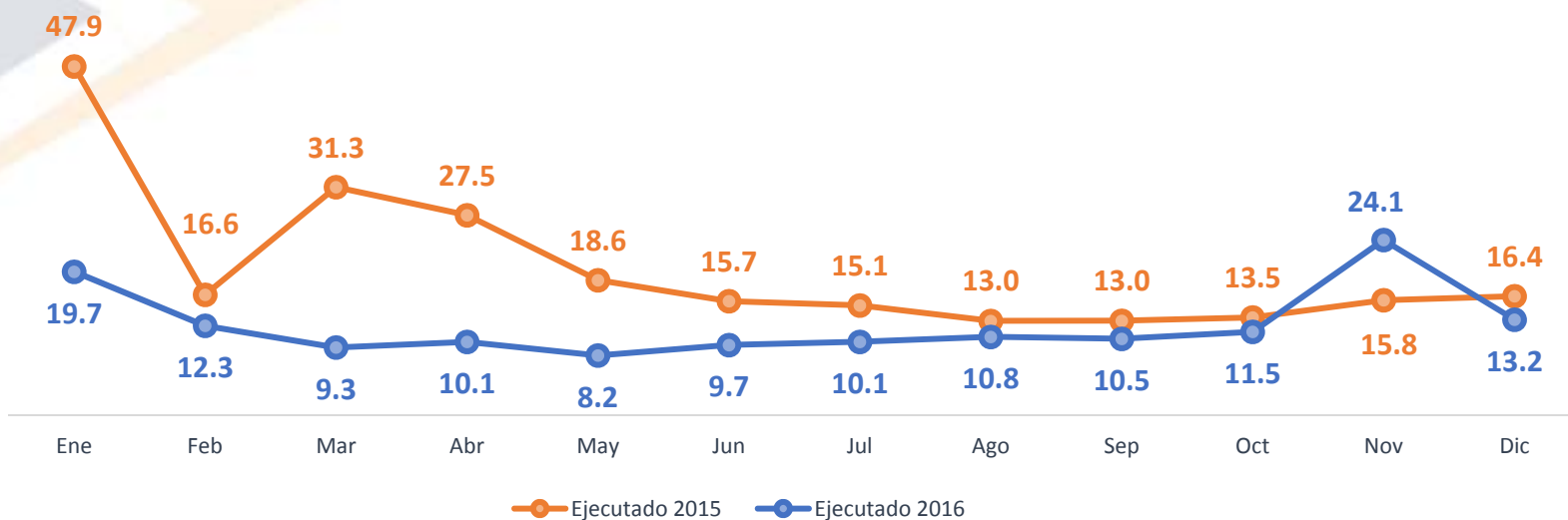
Precio Medio de Compra de Energía CDEEE 2015 - 2016 USCents/kWh
