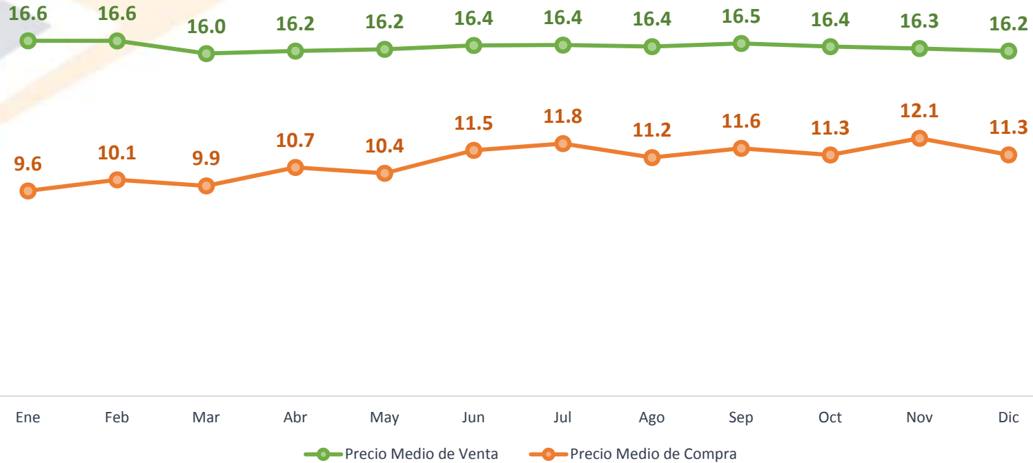
Precio Medio de Compra y Venta de Energía Edenorte Enero-Diciembre 2016 USCents/kWh
