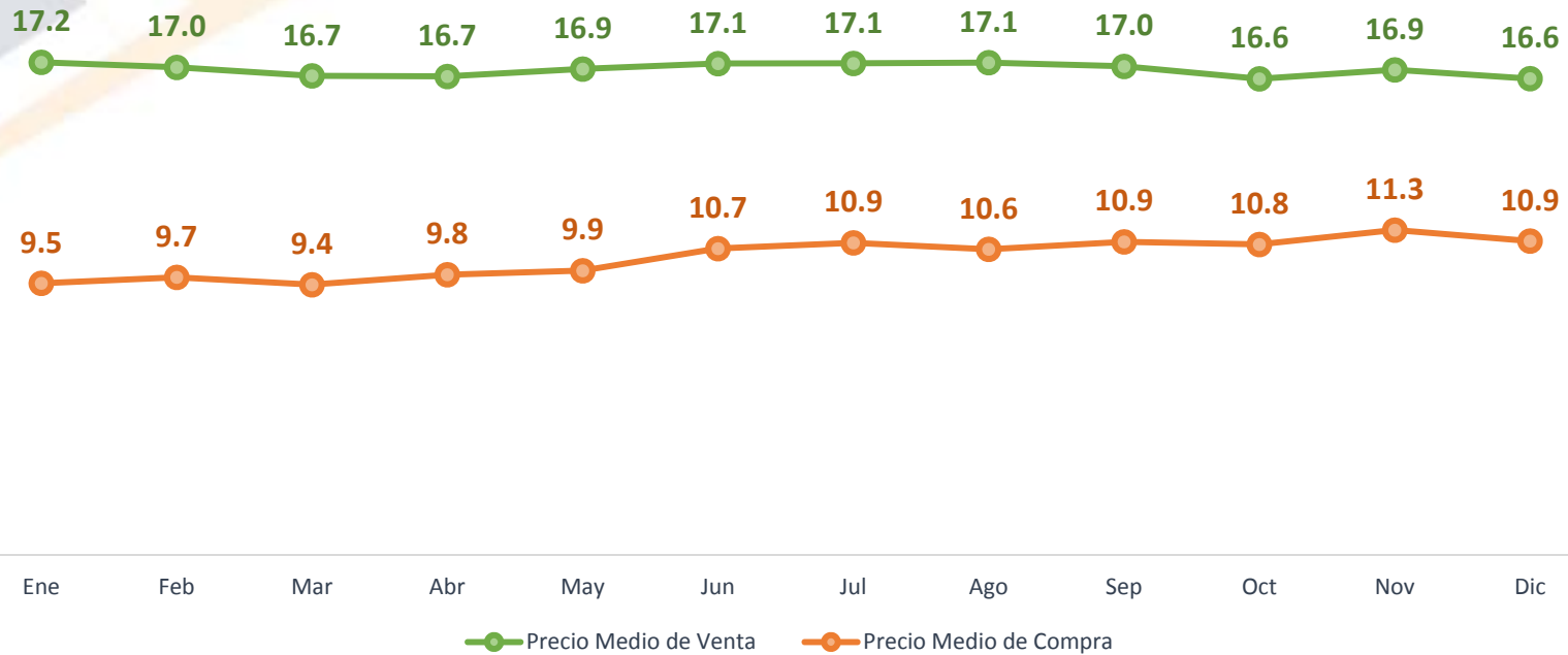
Precio Medio de Compra y Venta de Energía Total EDE's Enero- Diciembre 2016 USCents/kWh
