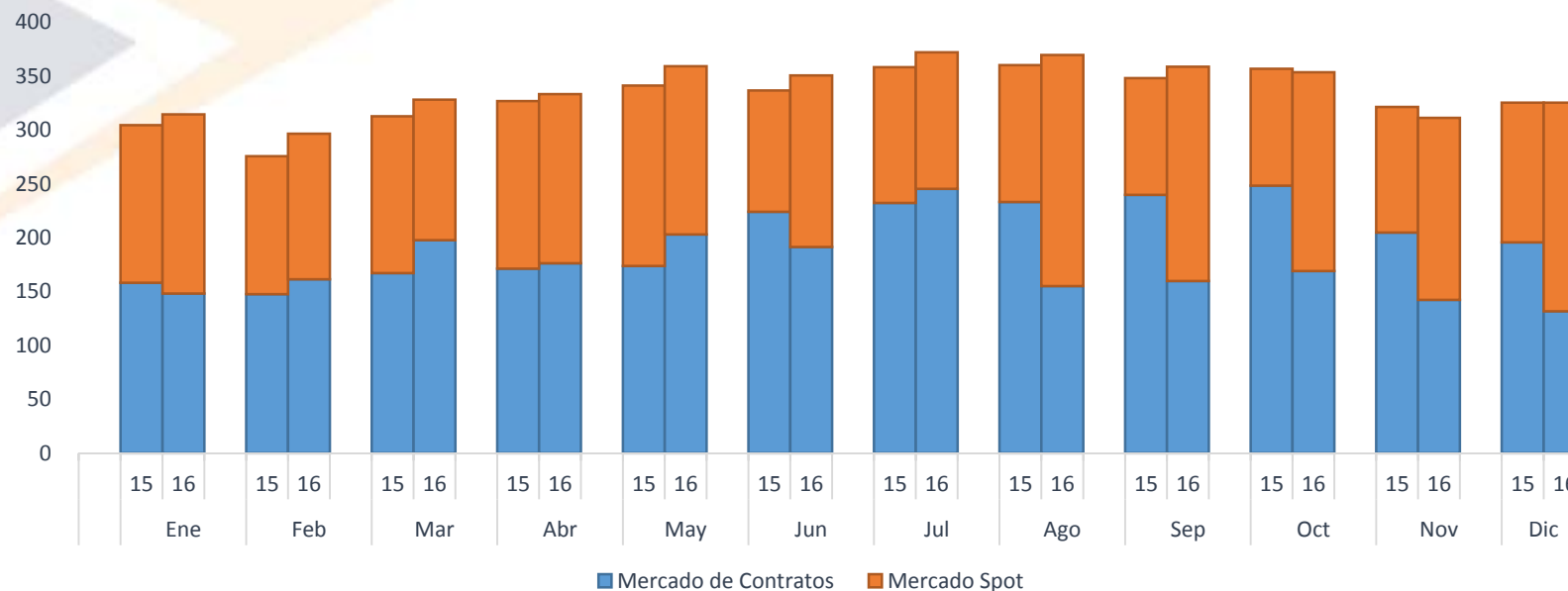
Compra de Energía por Mercado Edenorte 2015 - 2016 GWh
