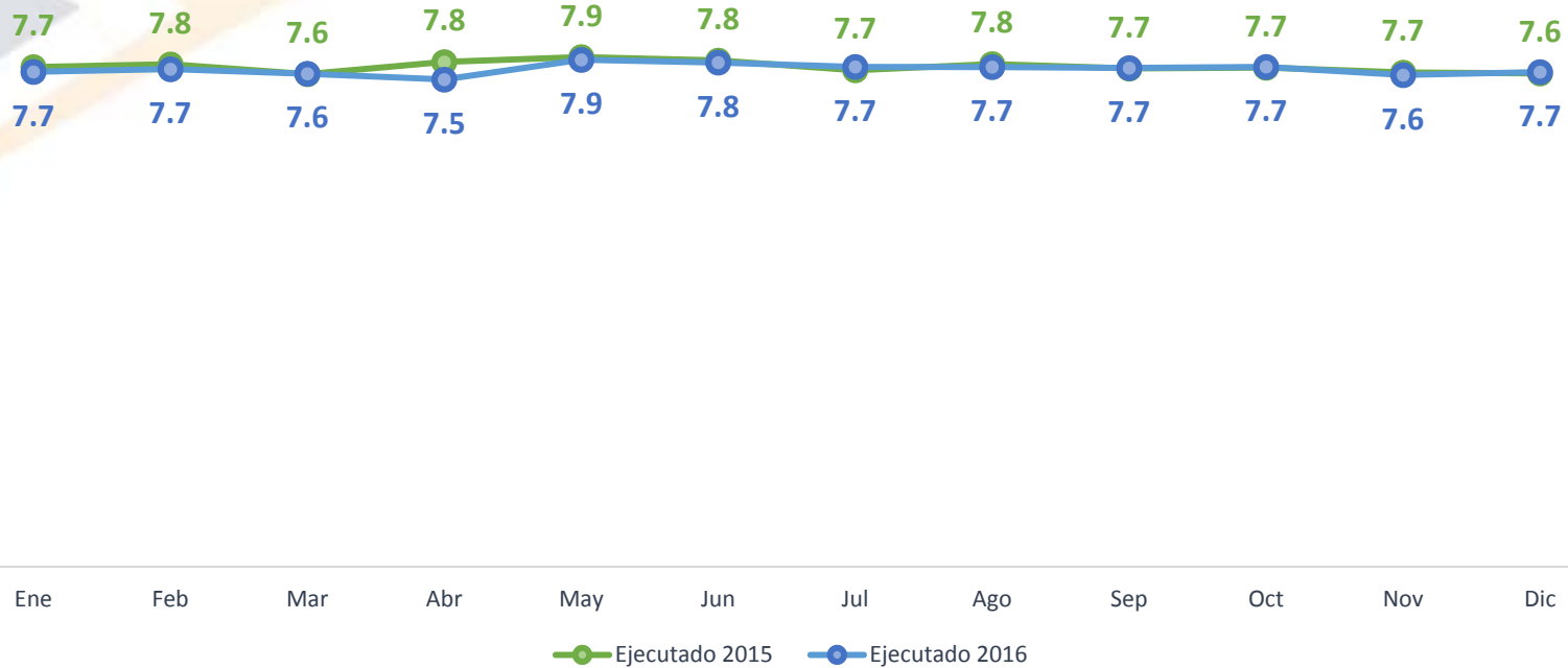
Precio Medio de Venta de Energía Edeeste 2015 - 2016 RD$/kWh
