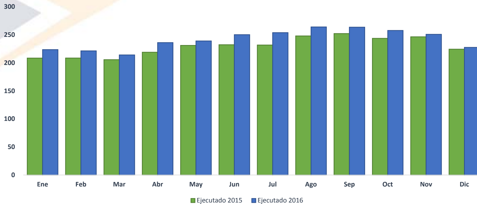
Energía Facturada Edenorte 2015 - 2016 GWh
