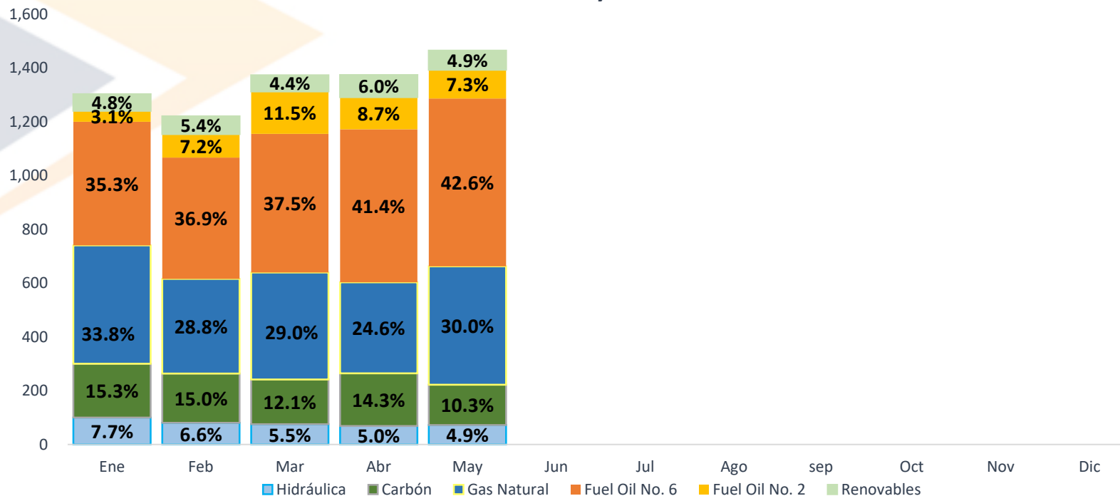
Generación de Energía por Tipo de Combustible 2019 GWh y %
